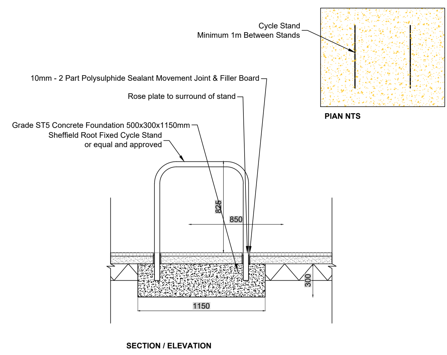
01 CYCLE STAND SCALE: 1:20 @ A1
