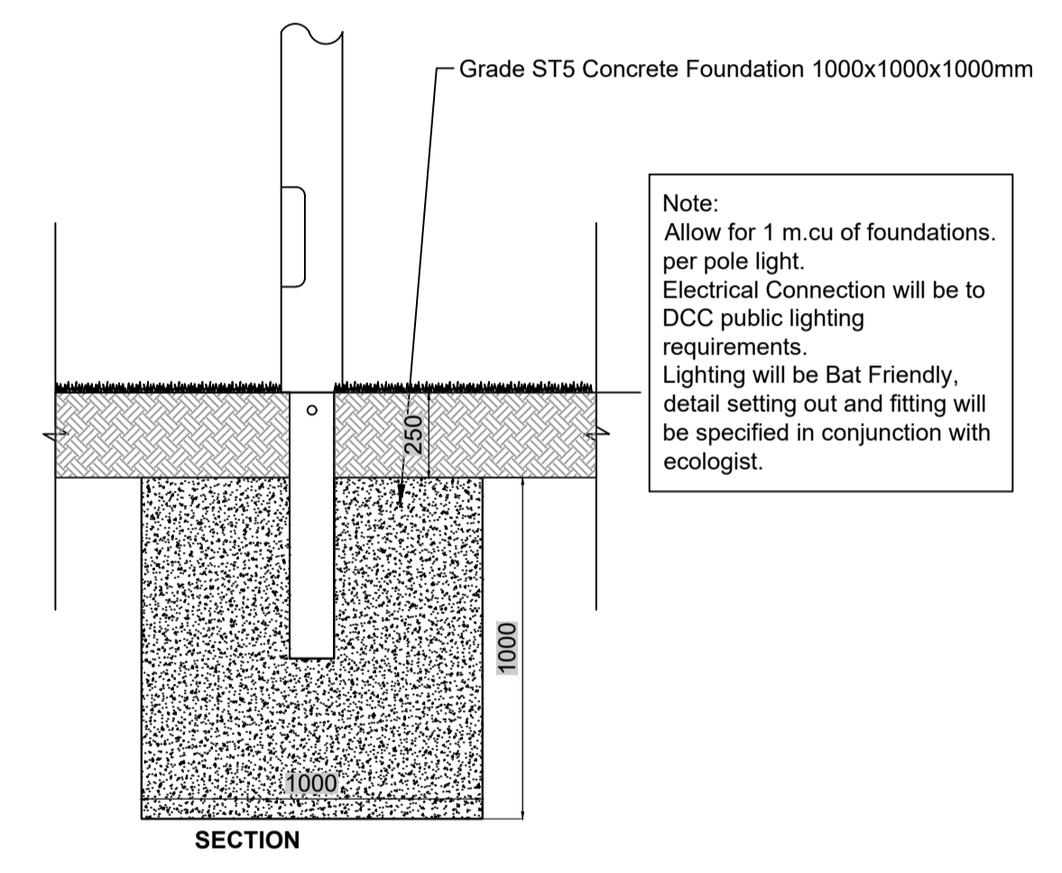
04 PATH POLE LIGHT SCALE: 1:20 @ A1
