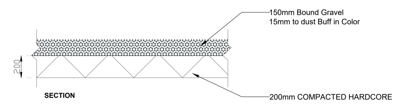
07 SELF BOUND GRAVEL SCALE: 1:20 @ A1
