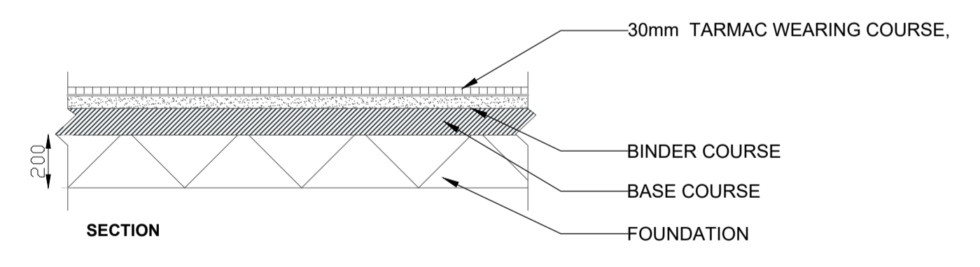
06 TARMAC DETAIL SCALE: 1:20 @ A1
