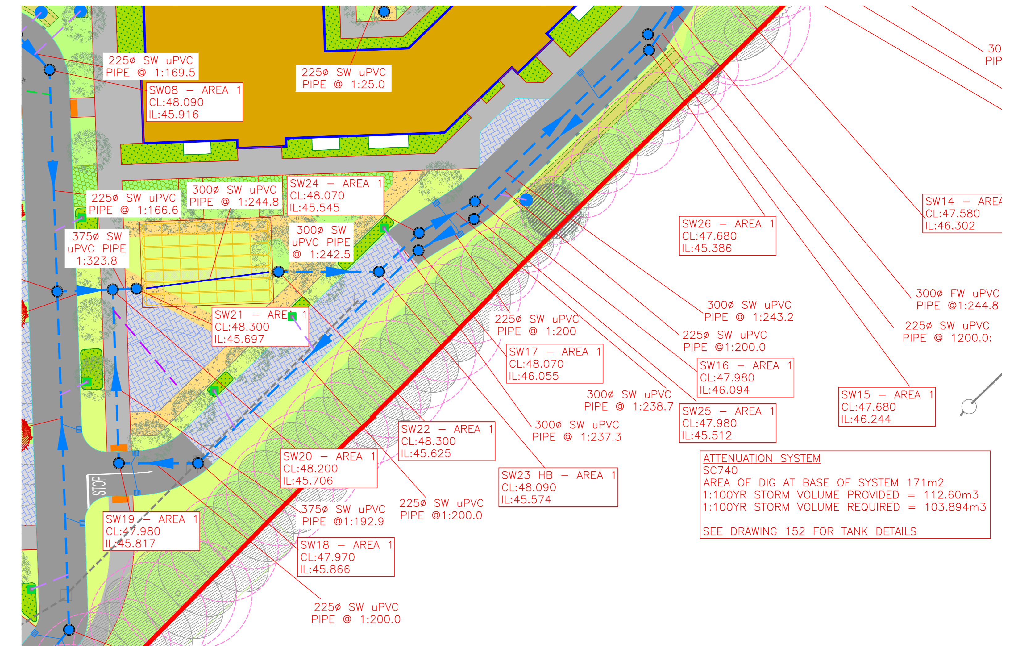
SITE LAYOUT SCALE N.T.S.
