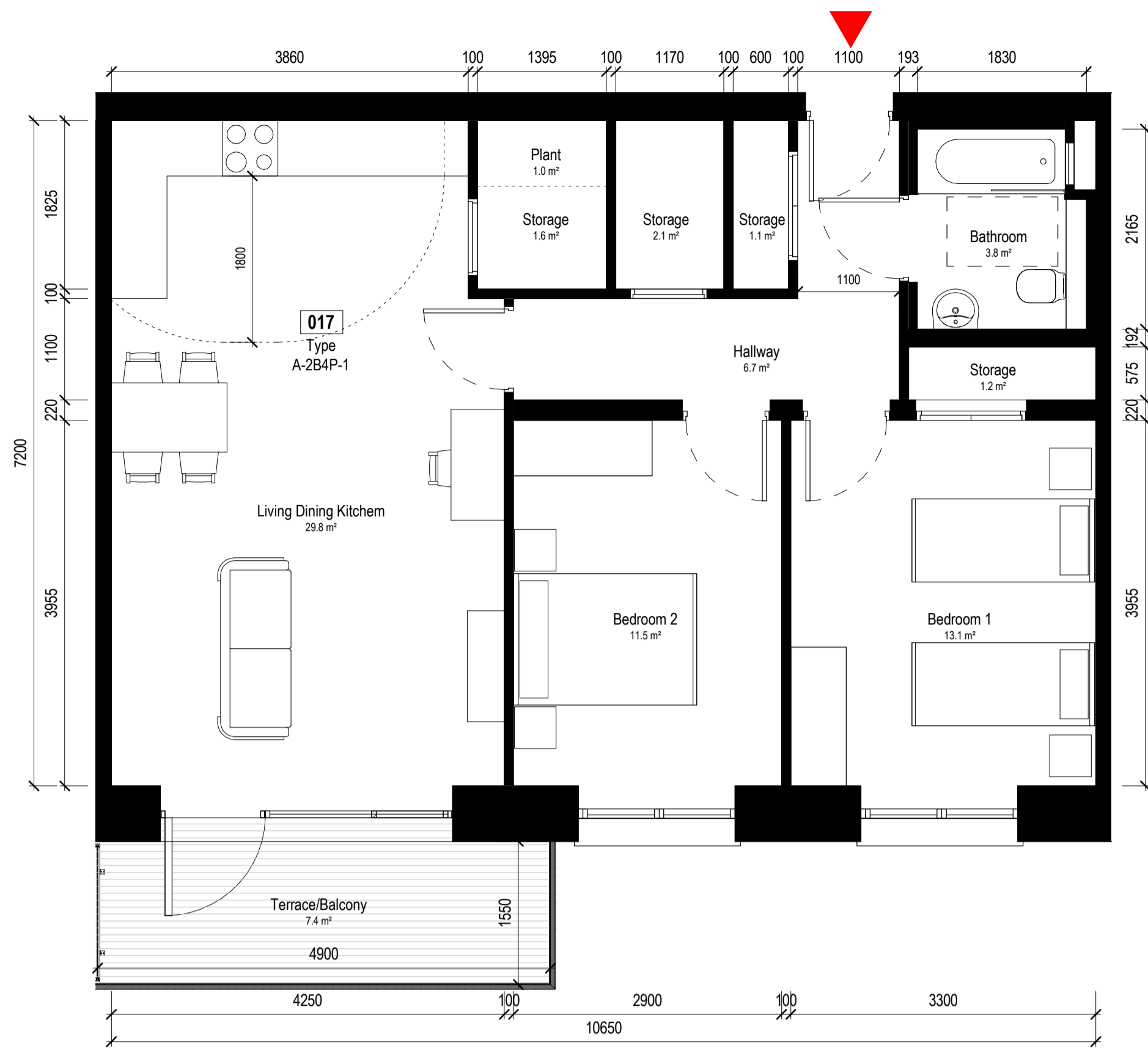
4 Type A-2B4P-1 1:50
