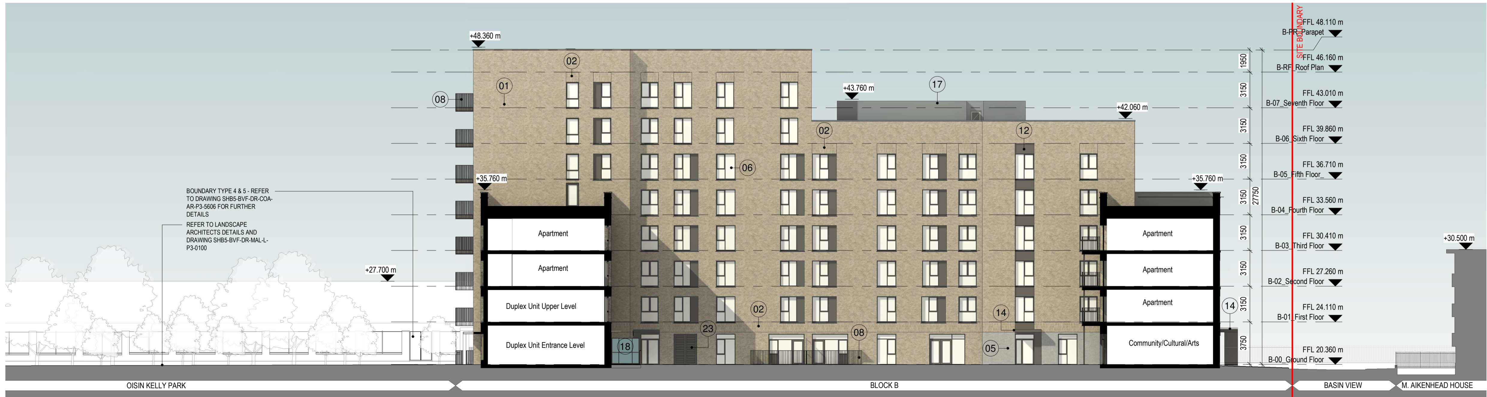
2 Section D-D 1:200
