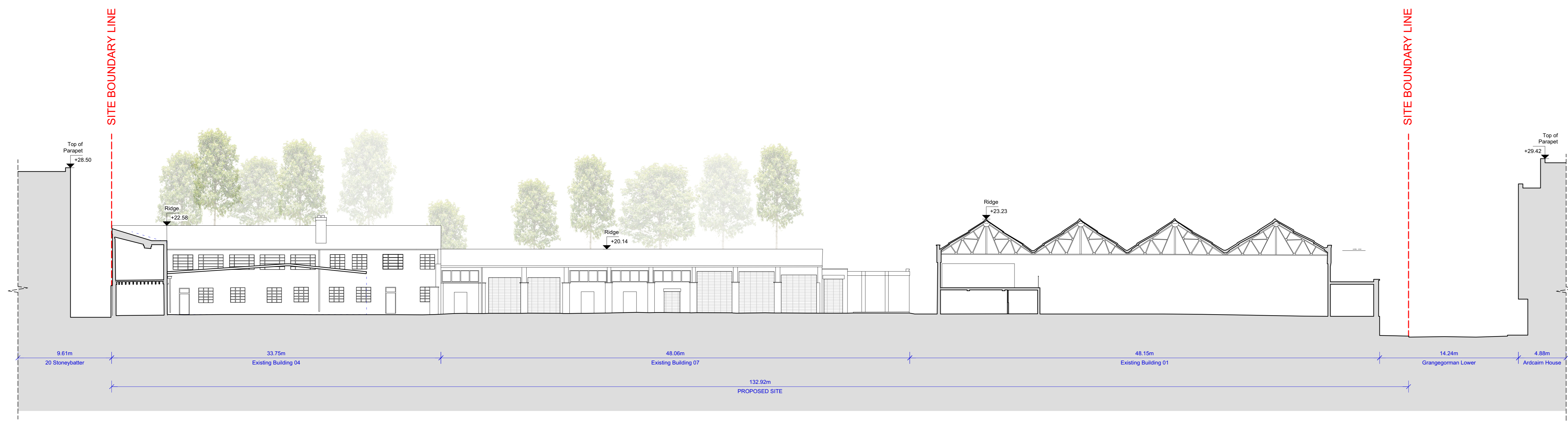
3 Existing Site Section Scale: 1:200
