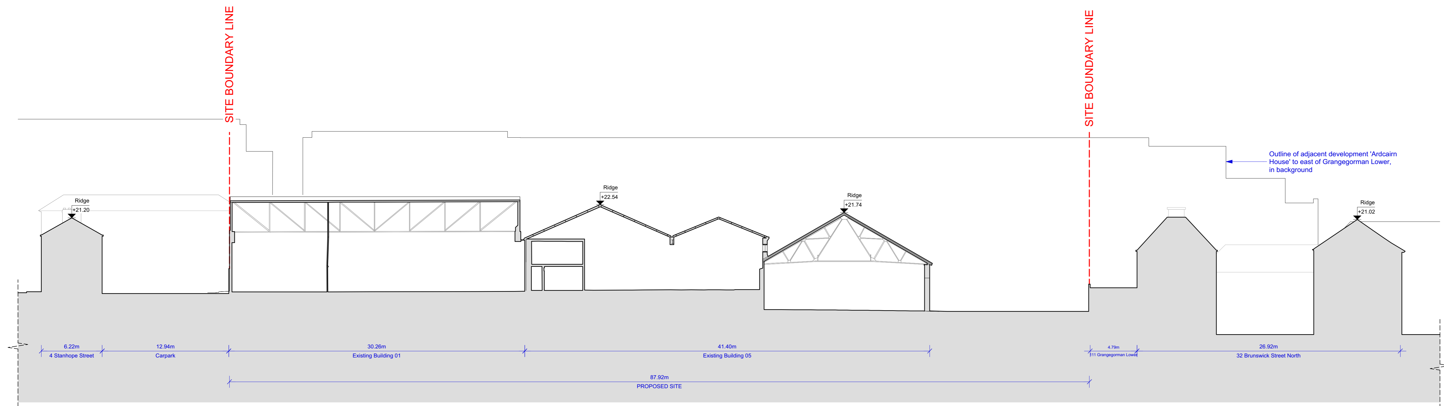
2 Existing Site Section Scale: 1:200
