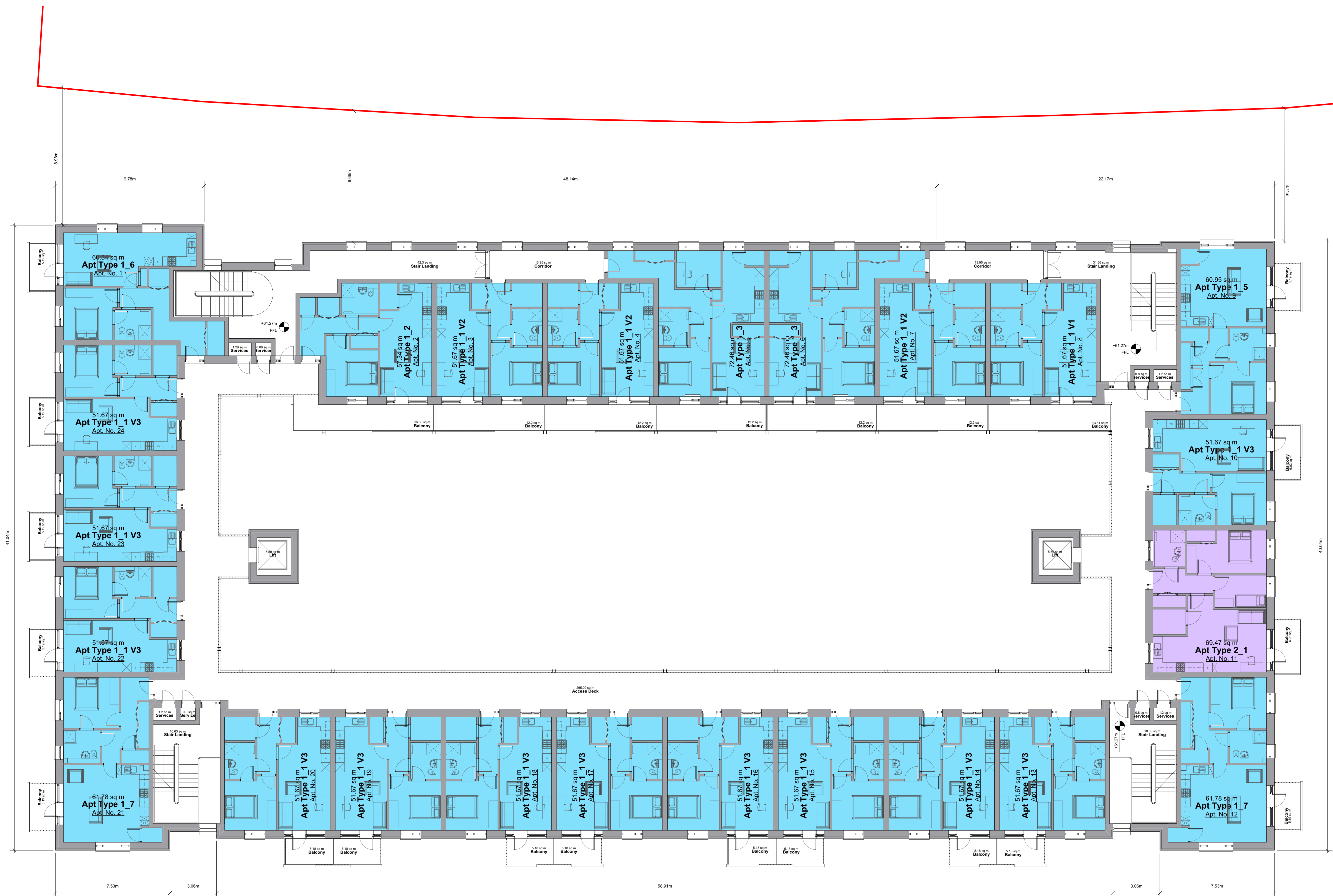
1 Floor Plan - Level +1 Scale: 1:100
