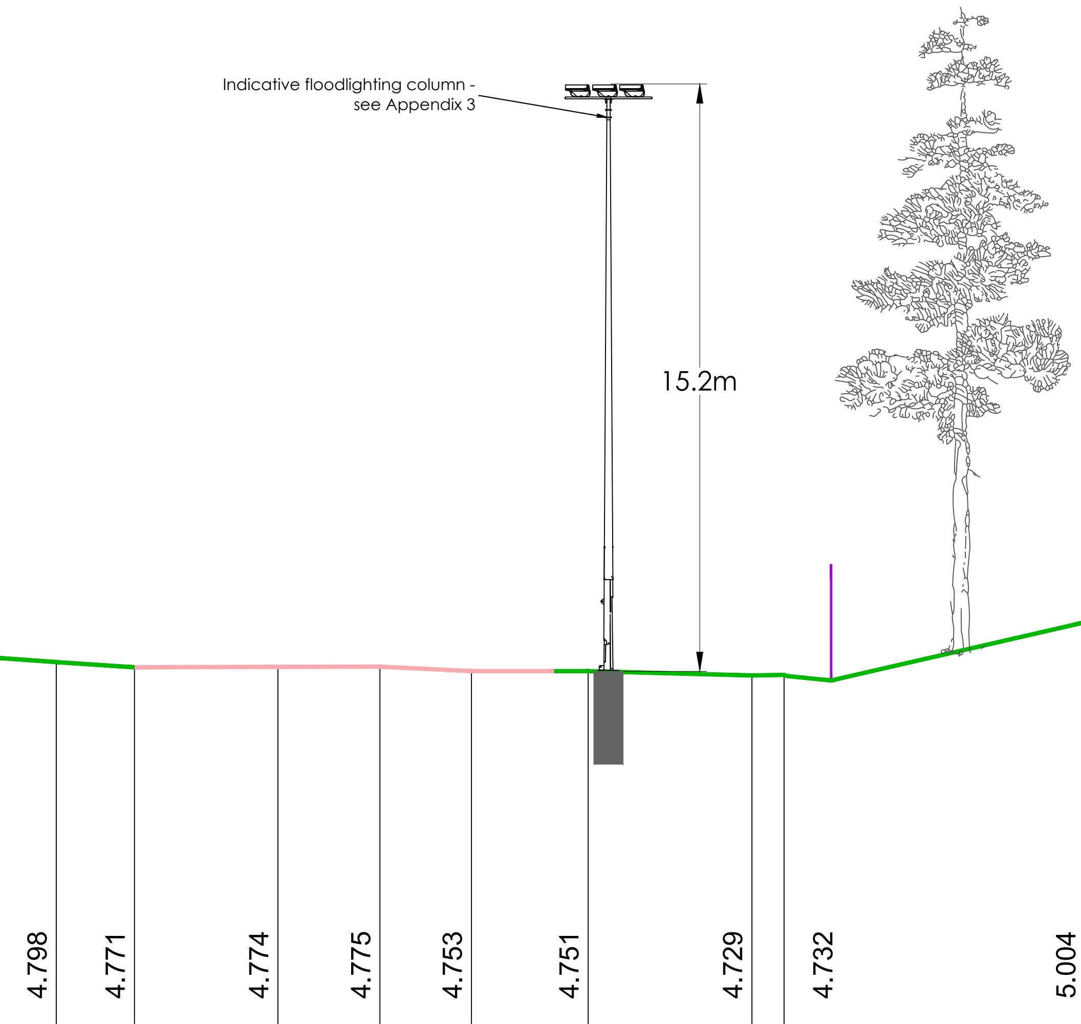
01 FLOODLIGHTING COLUMN SCALE: 1:100 @ A3
